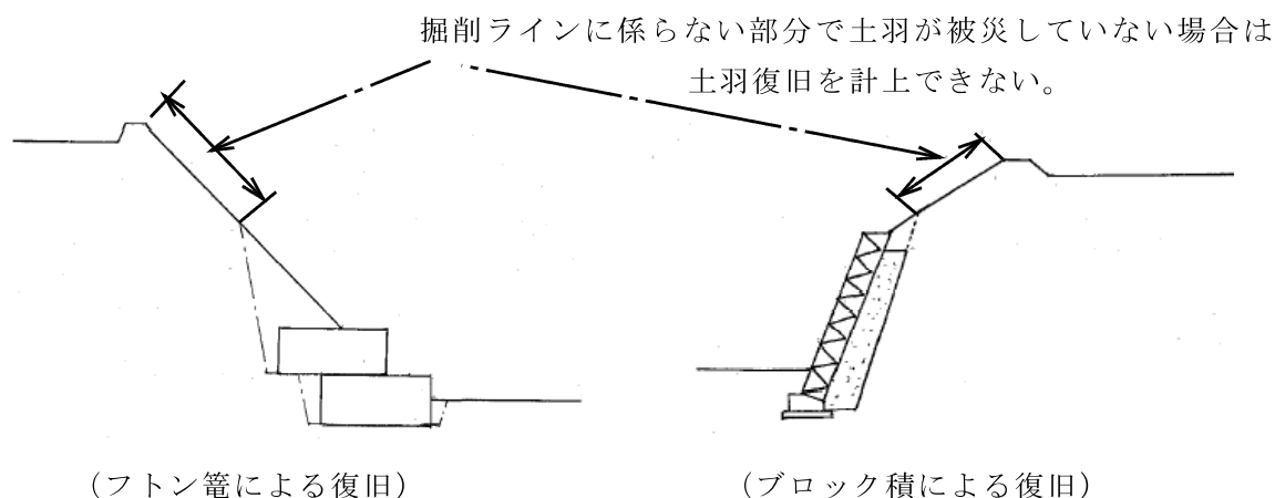
図－５：構造物を計画する場合
